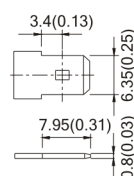
Клема T2
