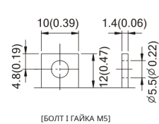
Клема B0
